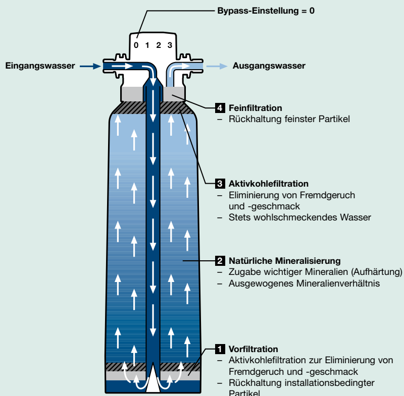
Aufbau einer BWT bestmin Filterkerze
